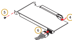
图2-9 显卡安装
