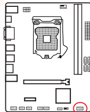
图2-5 F_PANEL1开机接口
