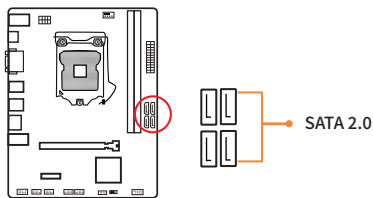
图2-10 SATA接口
