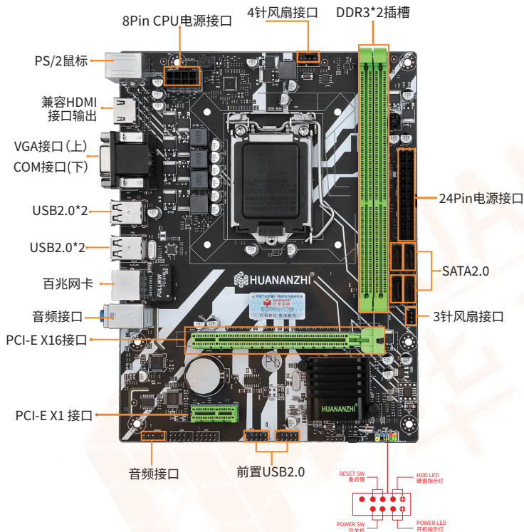
图1-1 H61 PLUS主板图解
